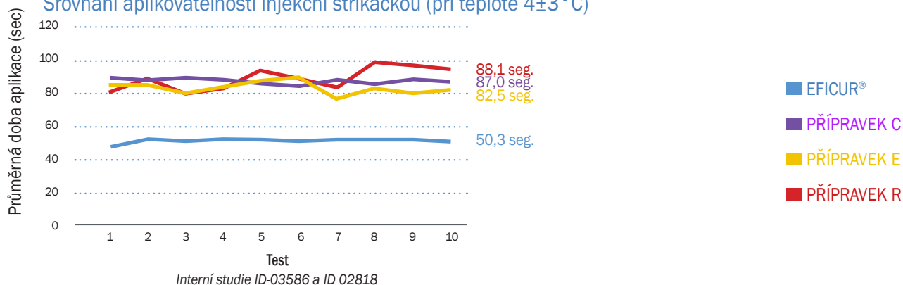
Porovnání viskozity
