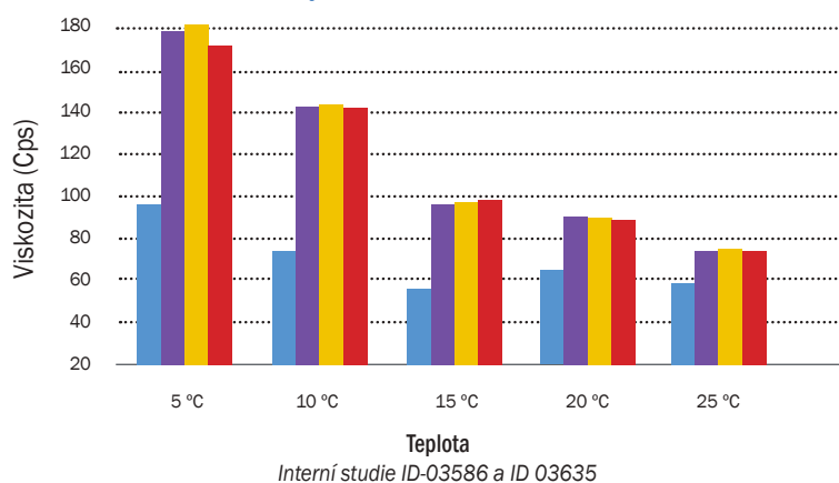
Porovnání viskozity
